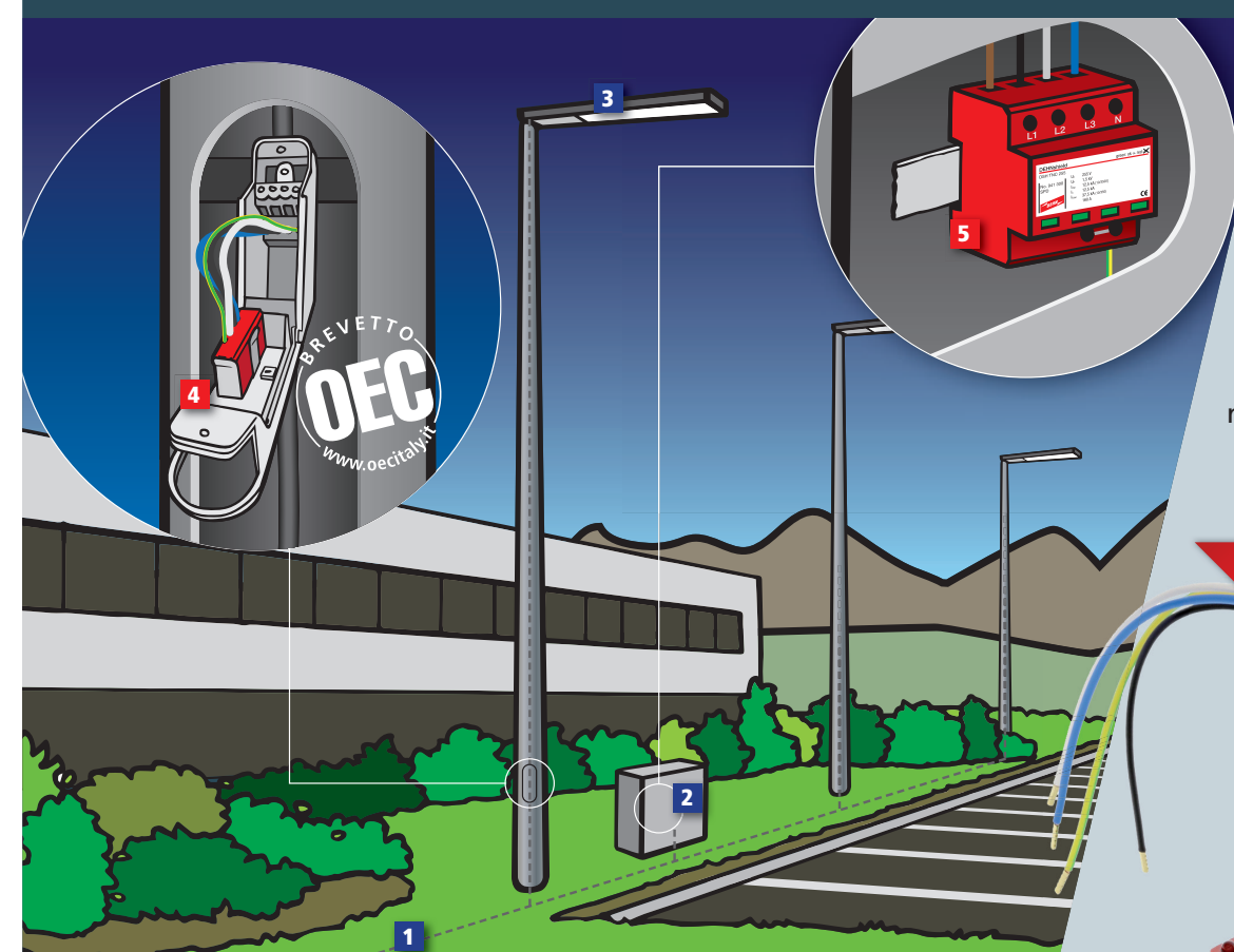
DEHNguard L 2P 275 SO IP Art. 900 448 Limitatore Tipo 2 in esecuzione compatta IP65, con funzione di interruzione dell'alimentazione in caso di fine vita.
